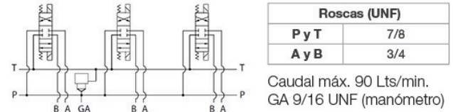
Circuito paralelo con válvula de alivio
